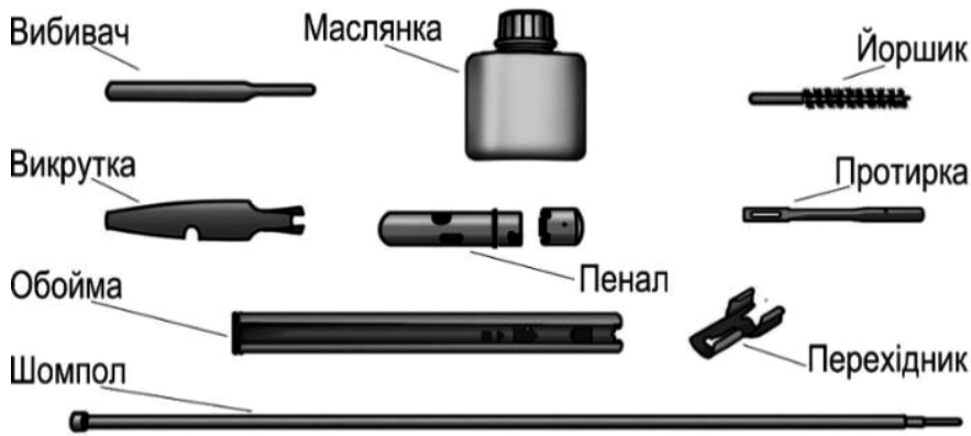
Лл. 18.3. Приладдя для чищення автомата АКС-74 (зберігається в сумці для магазинів)
