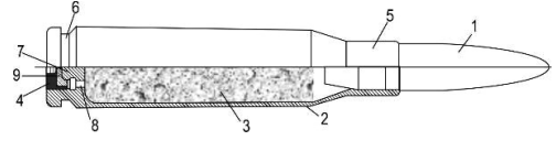
Іл. 22.3. Бойовий патрон: 1 — куля; 2 — гільза; 3 — пороховий заряд; 4 — капсуля; 5 — дульце; 6 — проточка; 7 — ковадло; 8 — затравочний отвір; 9 — ударний склад
